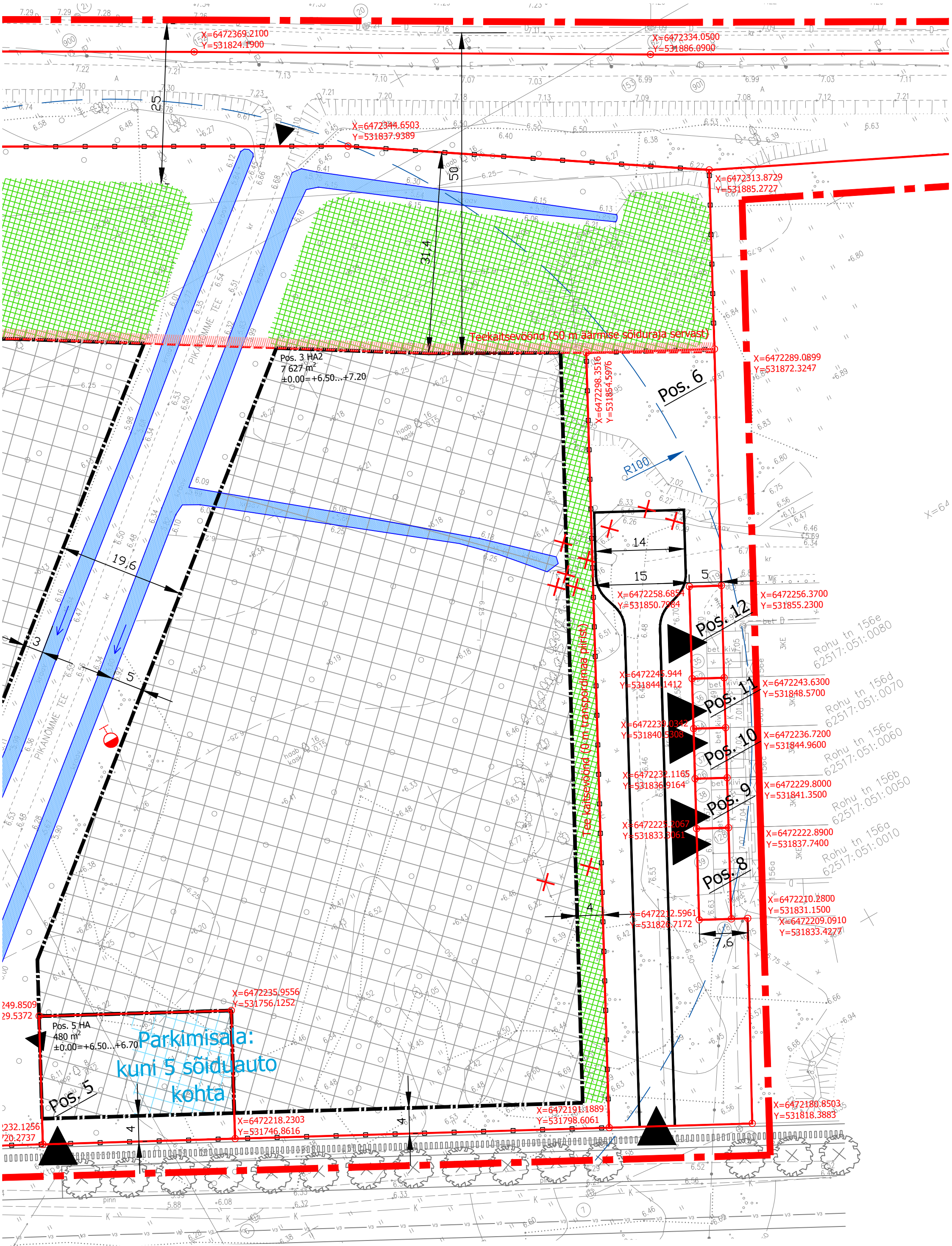
Niidu tn ja Ehitajate tee ristmiku (Ehitajate tee T8 kinnistu) lähiala detailplaneering Põhjoonise väljavõte M1: 500 (02.10.2017) OÜ Pärnu Instituut töö nr 15-04
