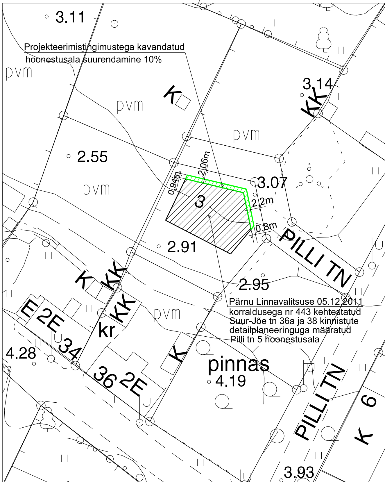
Lisa 1 projekteerimistingimused Pilli tn 5 Asendiskeem M 1:500
